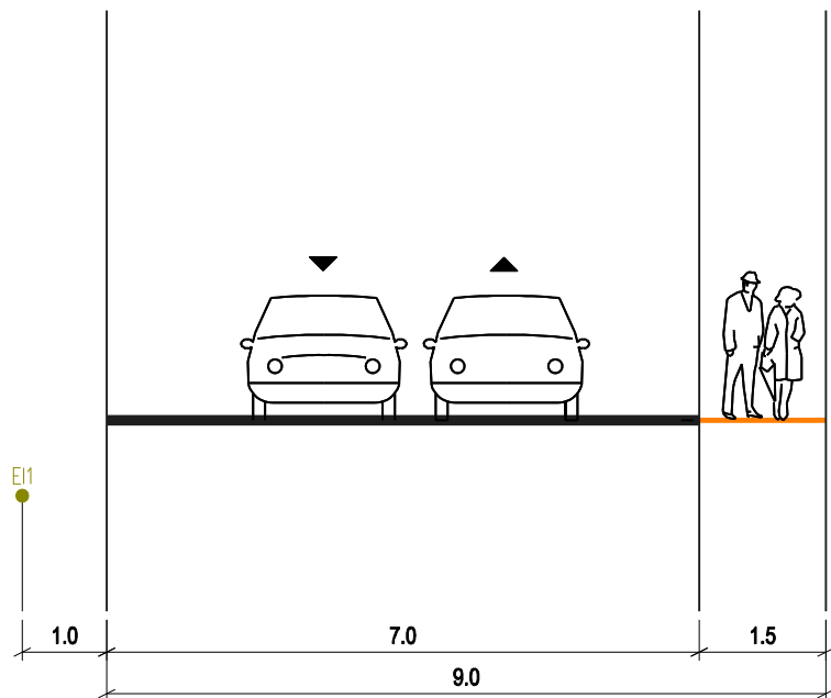
GRIEZUMS 1 - 1
