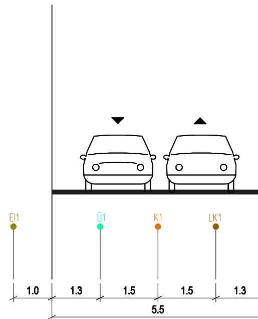
GRIEZUMS 2 - 2
